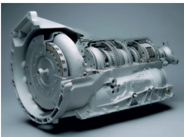
BMW X5 6-gang Automatikgetriebe
